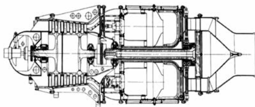
Двигун ТРД-1
